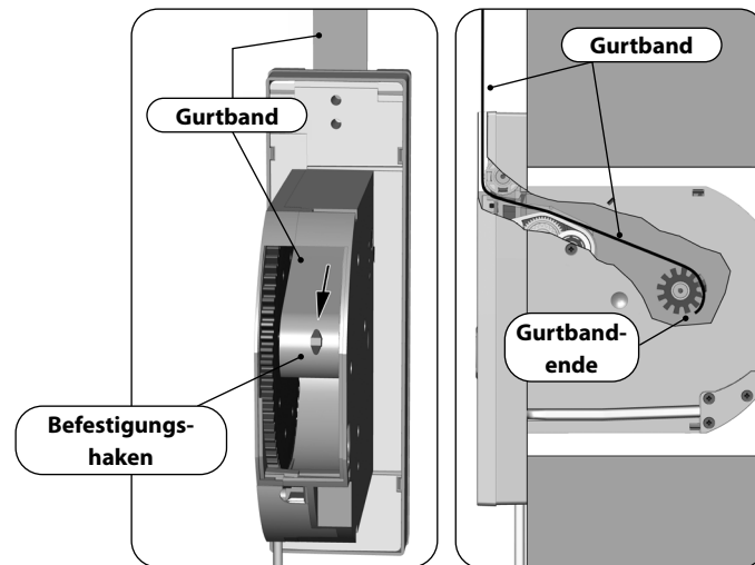
Gurtbandverlauf im RolloTron Standard DuoFern
