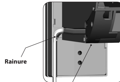
Dispositif anti-arrachement
